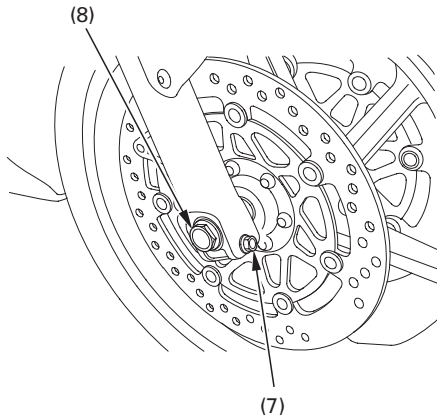
(7) Akselin kiristyspultit (8) Etuakselin pultti
