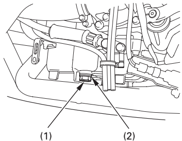
(1) Öljyn poistotulppa
