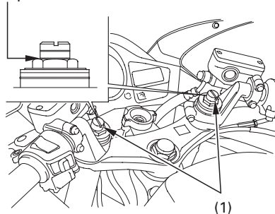
(1) Esijännityksen säätö
