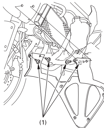
(1) Kiinnike A
